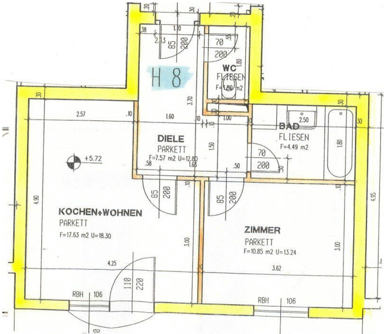
Grundriss
