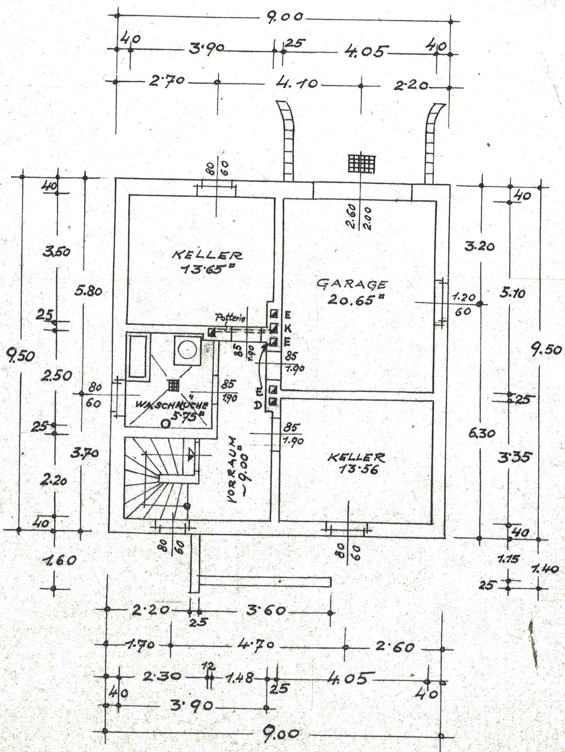
KELLERGESCHOSS
